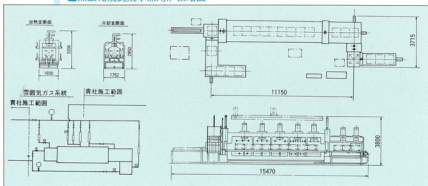
■無酸化焼鈍焼準兼用炉概略図
