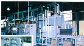
トレイプッシャー式連続無酸化焼鈍焼準兼用炉
